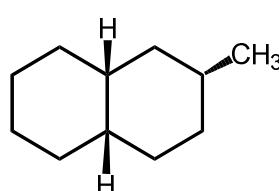
2 \alpha -метил- цис -декалин
