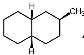
2 \beta -метил- транс -декалин
