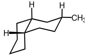
2 \beta -метил- транс -декалин
